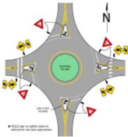
Mini Roundabout
